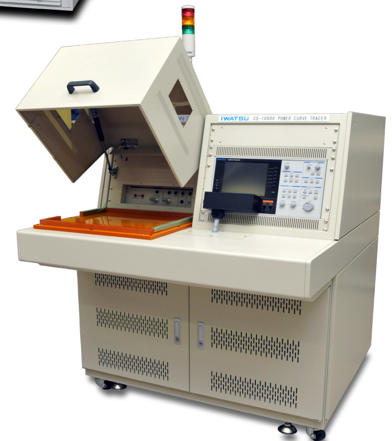
Curve Tracer model : CS-10800 CS-10400
